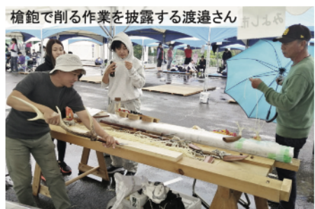
槍鉋で削る作業を披露する渡邊さん
